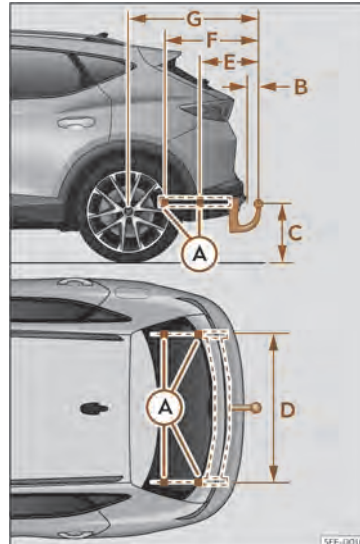
SI. 189 Mere in pritrilne točke za naknadno vgradnjo vlečne naprave
