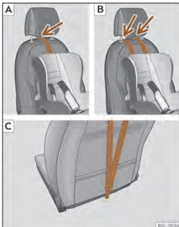
Sl. 30 Sovoznikov sedež: pritrдитеv s pasom Top Tether.
