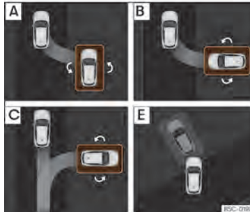
Sl. 179 Na zaslonu infotainment sistema: pregled načinov parkiranja.
