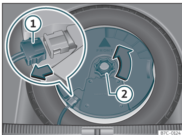
Sl. 198 V prtlačniku: demontaža globokotonskega zvočnika.
