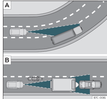
Sl. 154 [A] Vozilo v ovinku. [B] Spredaj vozeči motorist prehiteva zunaj območja dosegata radarskega senzorja.
