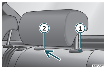
Sl. 99 Zadnji vzglavnik: demontaža
