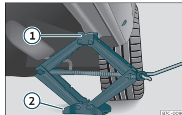
Sl. 39 Prečni nosilec: namestitev dvigalke.
