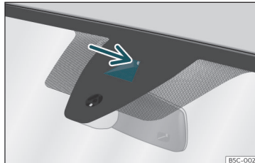
Sl. 142 V vetrobranskem steklu: vidno polje kamere asistencije za ohranjanje smeri na voznem pasu Lane Assist.
