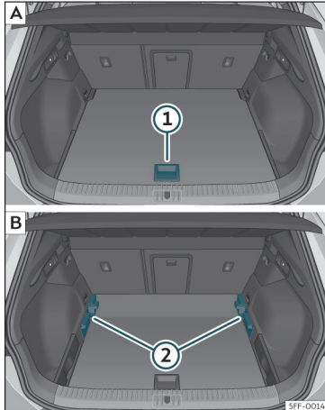
Sl. 109 Variabilno dno prtljažnika: A zgornji položaj; B spodnji položaj
