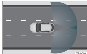
Sl. 144 Območje zaznavanja senzorjev. »»
