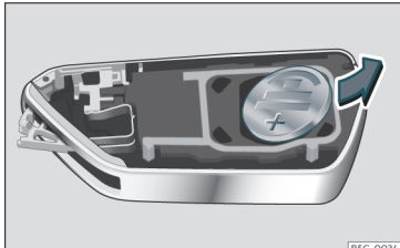
Sl. 69 Ključ vozila: odstranjevanje baterije.
