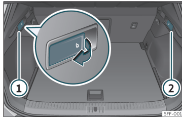
Sl. 103 V prtljažniku: ročici za sprostitve naslonjala zadnje sedežne klopi.
