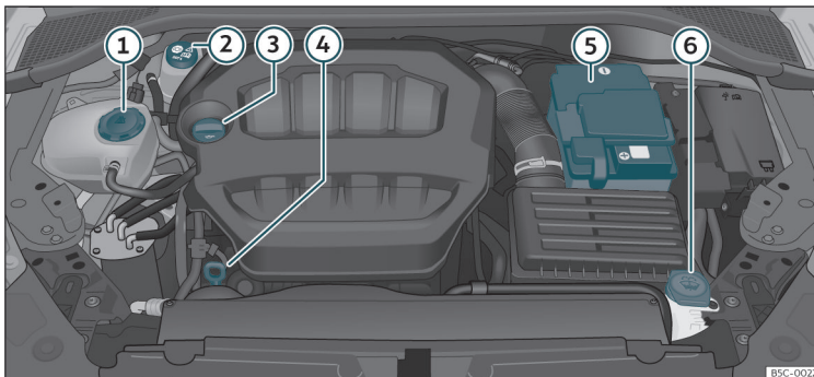
SI.185 Pregled položaja posameznih komponent
