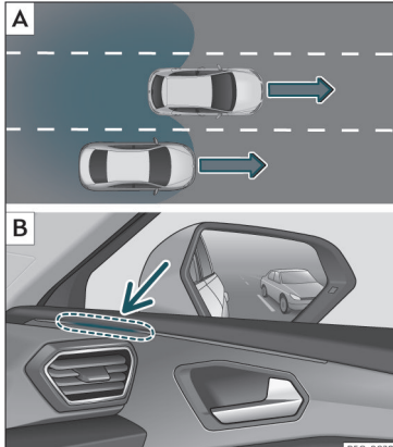
Sl. 163 Shematski prikaz: [A] Postopek prehitevanja na osrednjem pasu in nato menjava na desni vozni pas. [B] Prikaz asistencije za menjavo pasu s kontrolno lučko na desni strani.
