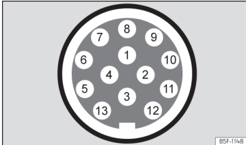
Sl. 178 Shematski prikaz: dodelitev konektorskih zatičev v električni vtičnici za prikolico.
