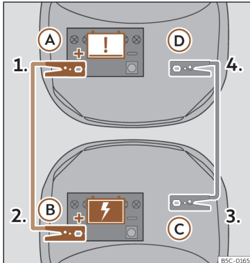
Sl. 42 Shema priklopa za vozila s sistemom start-stop.
