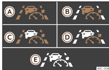
Sl. 166 Na zaslonu kombiniranega instrumenta: kontrolne lučke.
