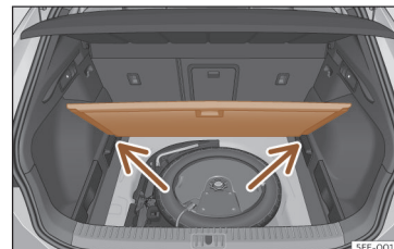
Sl. 116 Variabilno dno prtljažnika: v nagnjenem položaju
