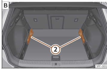
Sl. 115 Variabilno dno prtljažnika: [A] zgornji položaj; [B] spodnji položaj
