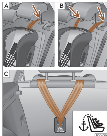
Sl. 29 Zadnji sedež: nastavev in vgradnja glede na pas Top Tether.
