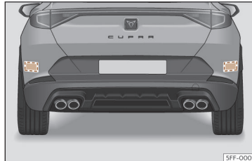
Sl. 151 Območje za vozilom: območja radarskih senzorjev.
