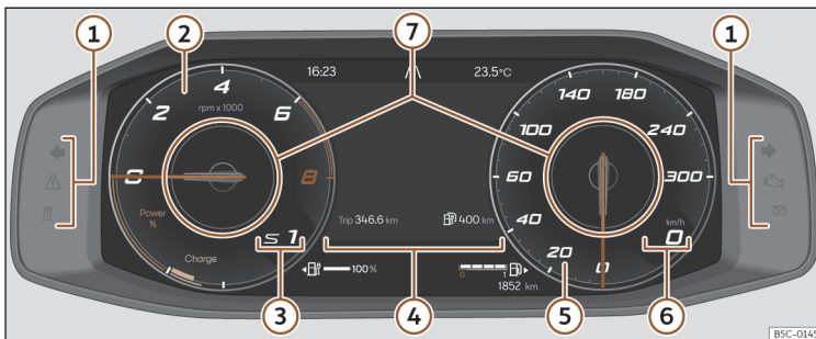
Sl. 52 Digitalni kombinirani instrument (Digital Cockpit) v armaturni plošči (običajni pogled).
