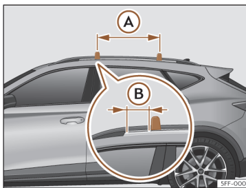
Sl. 123 Pritrdilne točke vzdolžnih nosilcev za strešni prtljažnik.
