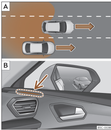
Sl. 171 Shematski prikaz: A ) Postopek prehitevanja na osrednjem pasu in nato menjava na desni vozni pas. B ) Prikaz asistencije za opozarjanje na vozila v mrtvem kotu s kontrolno lučko na desni strani.
