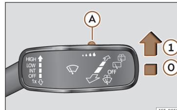
Sl. 97 Ročica za brisalce: nastavitve senzorja za dež A
