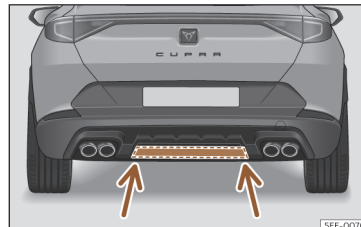
Sl. 86 Območje zaznavanja spodnjih senzorjev.
