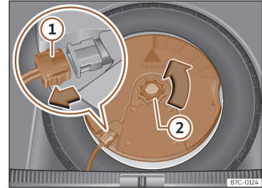
Sl. 224 V prtljažniku: demontaža globokotonskega zvočnika.
