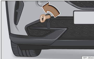
Sl. 44 Sprednji odbijač desno: privito vlečno uho.
