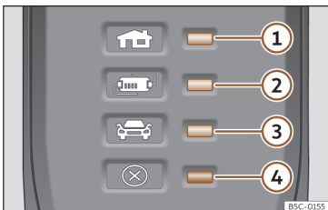
Sl. 200 Na polnilnem kablu za omrežne vtičnice: Kontrolna lučka za zaščitno napravo.
