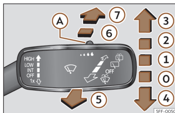
SI. 96 Upravljanje z brisalci vetrobranskega in zadnjega stekla
