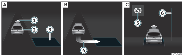
Sl. 181 Na zaslonu v kombiniranim instrumentu: prečno parkiranje. [A] Iskanje prostega parkirnega mesta. [B] Položaj za parkiranje. [C] Maneviranje.
