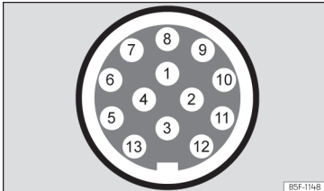
Sl. 186 Shematski prikaz: dodelitev konektorskih zatičev v električni vtičnici za prikolico.
