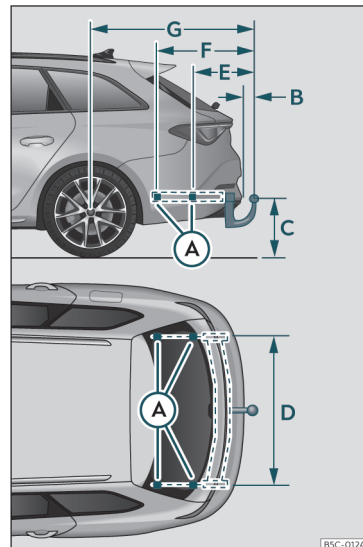
Sl. 188 Mere in pritrdilne točke za naknadno vgradnjo vlečne naprave
