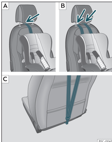
Sl. 30 Sovoznikov sedež: pritrditve s pasom Top Tether.
