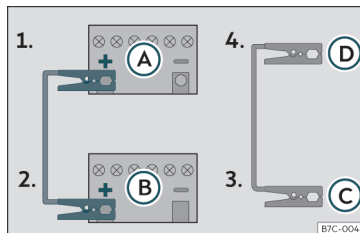
Sl. 42 Shema priklopa za vozila s sistemom start-stop.
