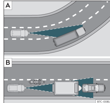
Sl. 162 [A] Vozilo v ovinku. [B] Spredaj vozeči motorist prehiteva zunaj območja doseg radarskega senzorja.
