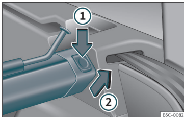
Sl. 122 V prtljajniku: odstranjevanje predelne mreže.
