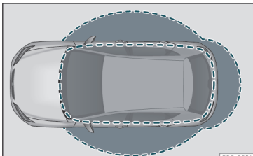
Sl. 76 Sistem zaklepanja in zagona brez ključa Keyless Access: območja približevanja
