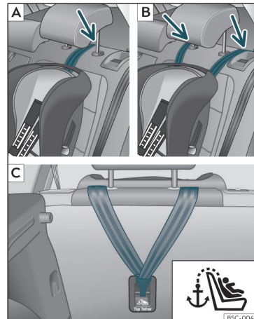
Sl. 29 Zadnji sedež: nastavitve in vgradnja glede na pas Top Tether.
