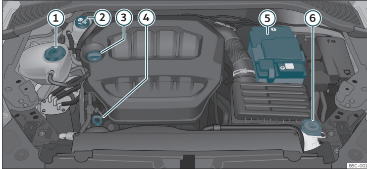
SI. 203 Pregled položaja posameznih komponent
