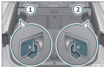
Sl. 107 V prtljajniku: ročici za sprostitve naslonjala zadnje sedežne klopi.
