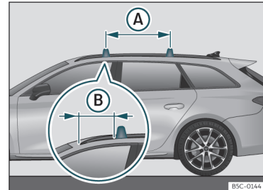
Sl. 125 Pritrdilne točke vzdolžnih nosilcev za strešni prtljažnik.
