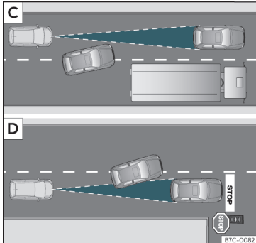
Sl. 163 [C] Vozilo menja vozni pas. [D] Eno vozilo zavija, drugo miruje.
