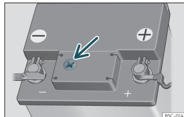
Sl. 210 Vidno okence na zgornji strani 12-voltnega akumulatorja (shematski prikaz).
