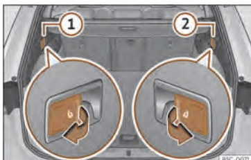
Sl. 113 V prtljažniku: ročici za sprostitev naslonjala zadnje sedežne klopi.
