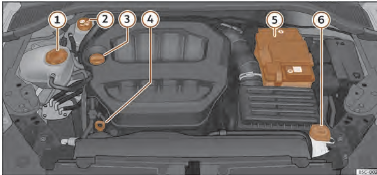
SI. 217 Pregled položaja posameznih komponent
