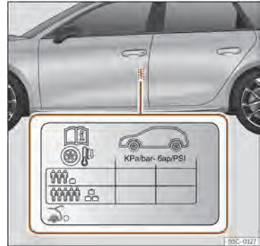
Sl. 229 Mesto vgradnje nalepke za tlak v pnevmatikah.
