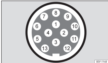
Sl. 187 Shematski prikaz: dodelitev konektorskih zatičev v električni vtičnici za prikolico.
