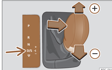
Sl. 138 Sredinska konzola: prestavljanje v načinu tiptronic
