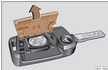
Sl. 67 Ključ vozila: odpiranje pokrova predalčka za baterijo.
