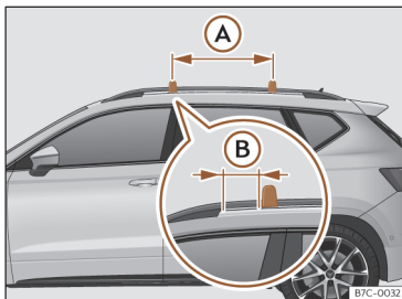
Sl. 118 Pritrdilne točke vzdolžnih nosilcev za strešni prtljažnik.
