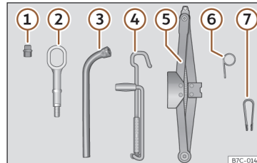
SI. 30 V prtljažniku pod dnom prtljažnika: avtomobilsko orodje.
