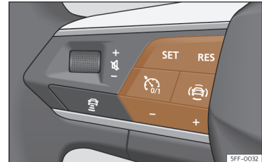
Sl. 150 Na večfunkcijskem volanu: tipke za upravljanje omejevalnika hitrosti.
