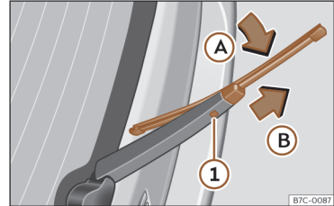
Sl. 39 Menjava metlice brisalca zadnjega stekla
