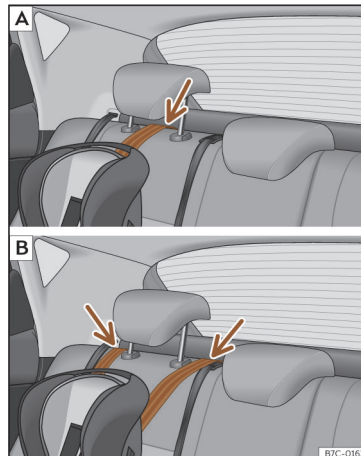
Sl. 27 Zadnji sedež: nastavitve in vgradnja glede na pas Top Tether. »
