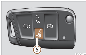
Sl. 66 Ključ vozila z alarmno tipko.
