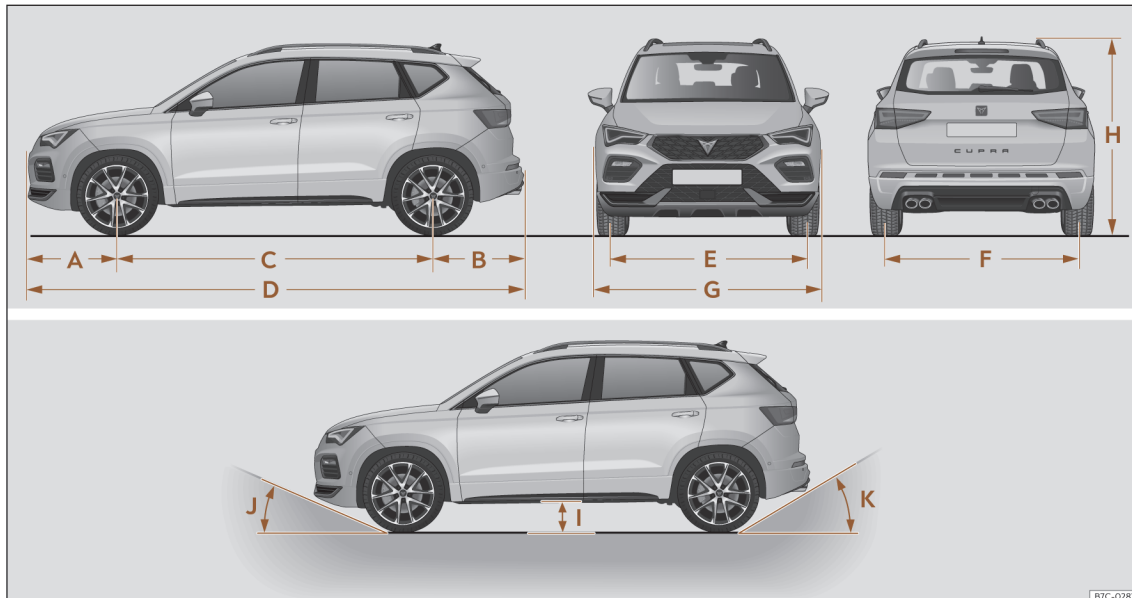
Sl. 210 Mere in koti
