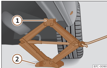
Sl. 36 Prečni nosilec: namestitev dvigalke.
