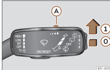
Sl. 92 Ročica za brisalce: nastavev senzorja za dež (A)
