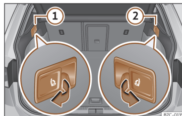
Sl. 103 V prtljažniku: vzvod za daljinsko sprostitvev levega (1) in vzvod za daljinsko sprostitvev desnega (2) naslonjala zadnjih sedežev.
