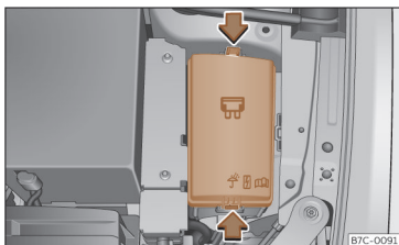
Sl. 47 V motornem prostoru: pokrov postaje z varovalkami.
