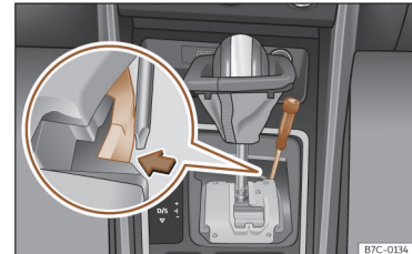
Sl. 140 Izbirna ročica: zasilno odklepanje zapore za premik ročice iz parkirnega položaja.
