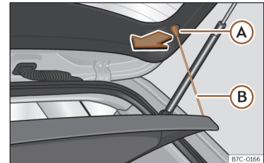
Sl. 105 V prtljažniku: odstranjevanje in nameščanje zadnje police
