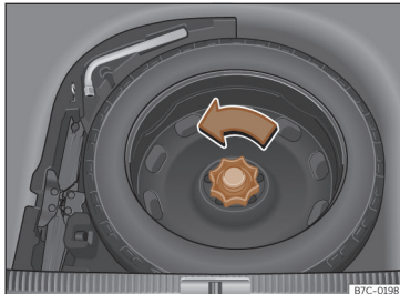
Sl. 208 V prtljažniku: dvignjeno dno prtljažnika.
